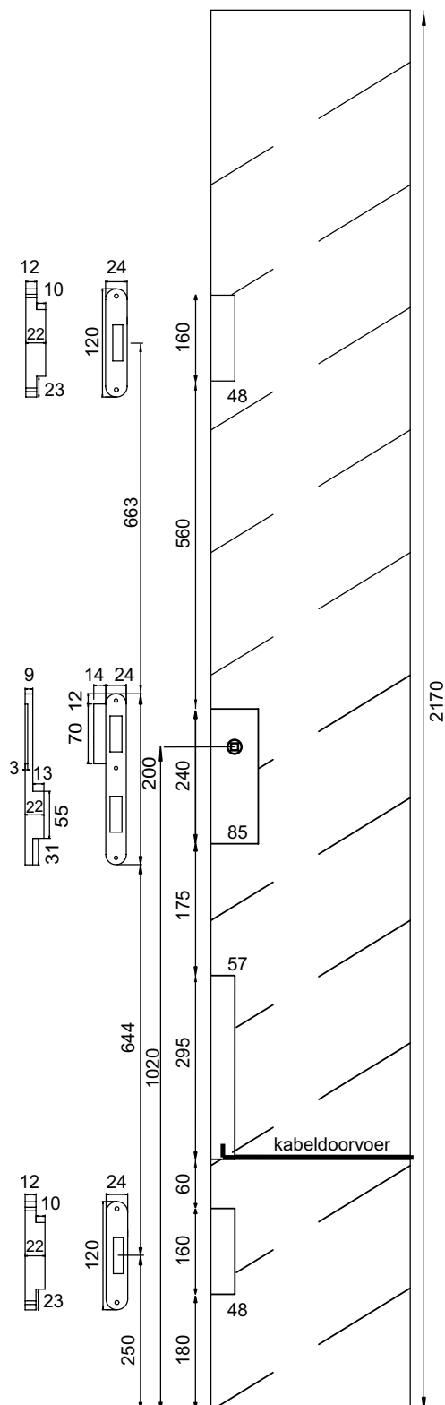
FREES AFSTANDEN
