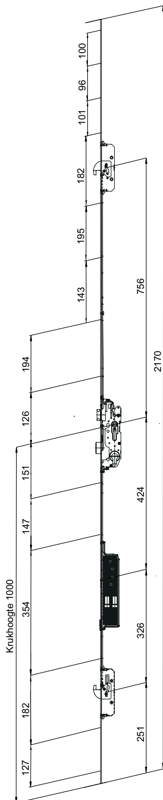
AFMETINGEN
