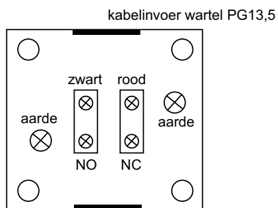
kabelinvoer wartel PG13,5
